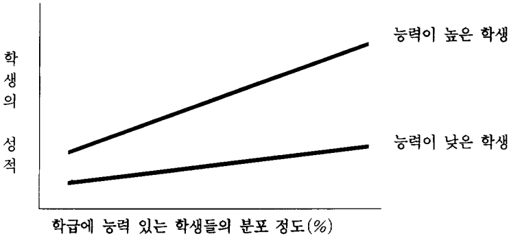
그림1 다차원효과와의 예시
